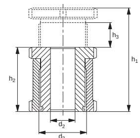
Precision levellers
